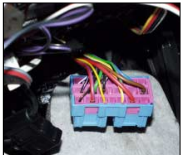
Sicht auf den Stecksocket von hinten
