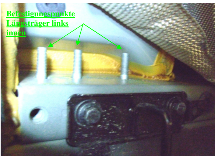
Befestigungspunkte Längsträger links innen nach Montage
