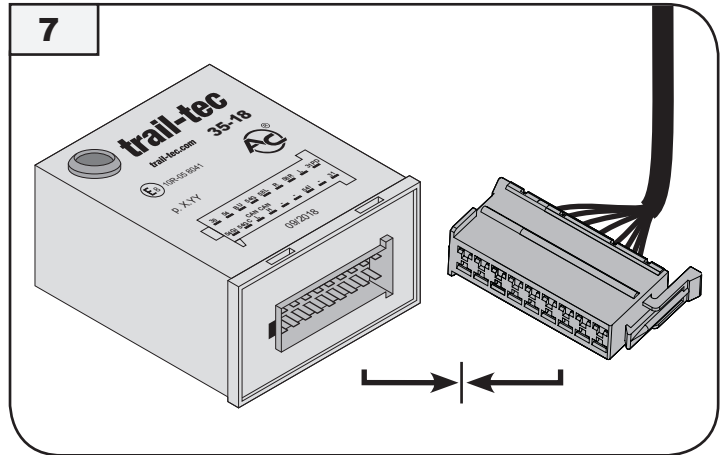
Modul Trail-tec 35-18 → Stecker 18 pin E-Satz modul Trail-tec 35-18 → socket 18 pin e-kit
