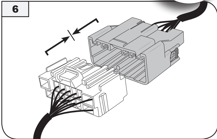
E-Satz Stecker → Fahrzeug Stecker e-kit socket → car socket
