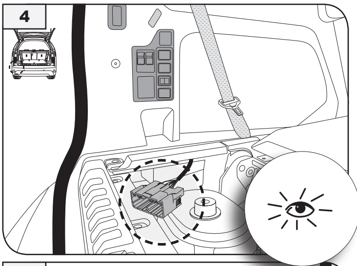
Fahrzeug Stecker car socket
