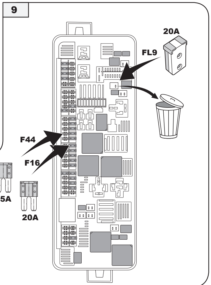
Sicherung 15A → Kammer F44, Sicherung 20A → Kammer F16, Sicherung 20A → Kammer FL9 fuse 15A → fuseslot F44, fuse 20A → fuseslot F16, fuse 20A → fuseslot FL9
